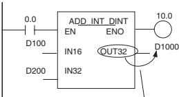
OUT32为DINT变量。因此，变量值传至D1000和D1001。
